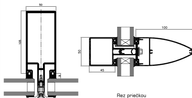
Rez priečkou
