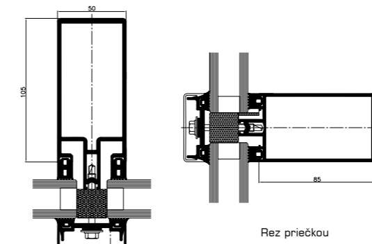
Rez stĺpikom
